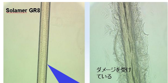
水酸化 Na による毛髪の膨潤テスト
