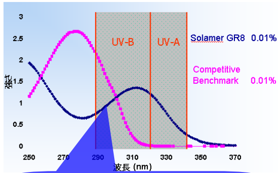
Solamer GR8 の UV スペクトル
